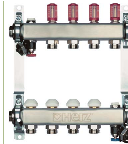
Rys. 5. Rozdzielacz HERZ 8632 ze stali szlachetnej
